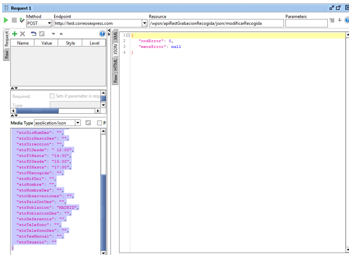
Ilustración 4 – Nuevo proyecto REST con SOAPUI – Modificar recogida
